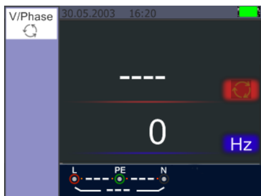
Startbild der Phasensequenzmessung
